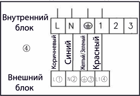
④ Диаграмма соединения для моделей 24, 30 (модели на охлаждение)
