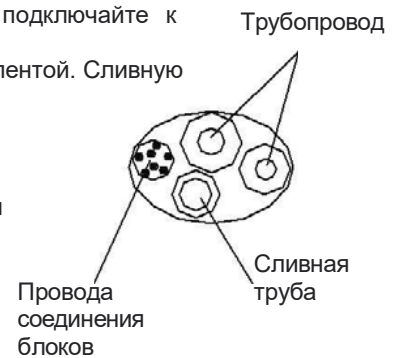
Рис.6 монтажная панель.
