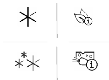
Fig. 10 Программные опции
