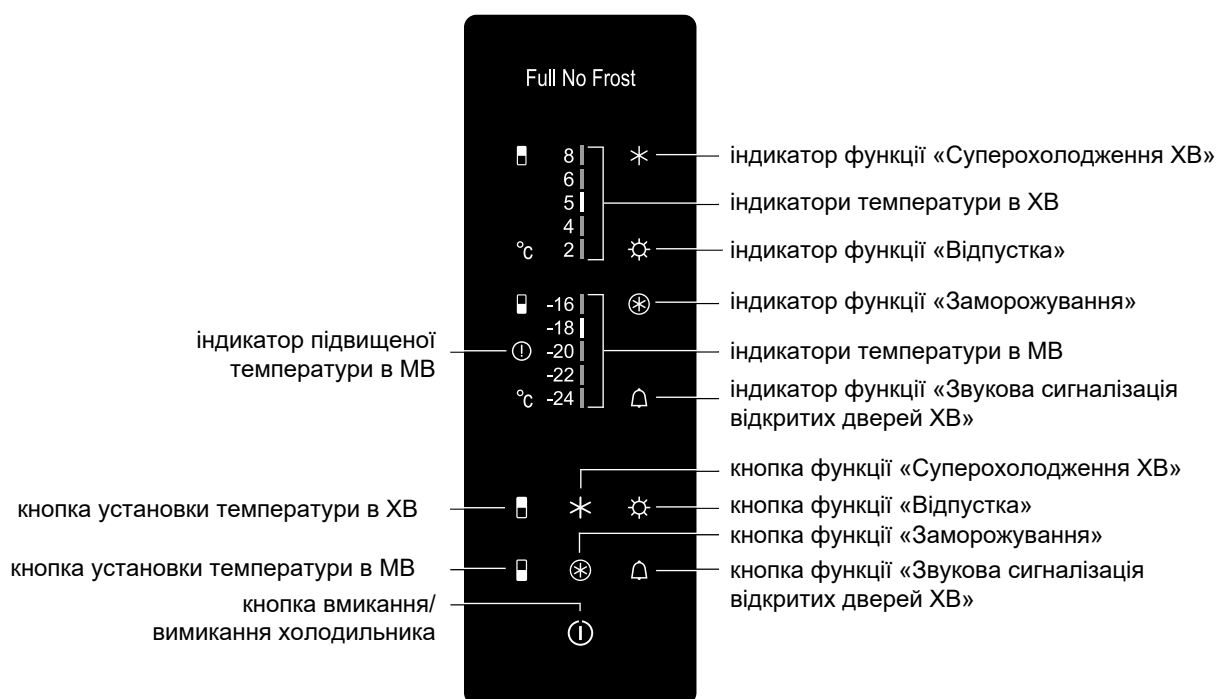
Рисунок 3 — Блок управління
