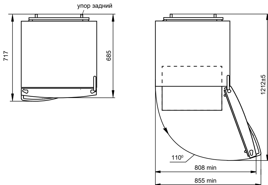
Рисунок 2 — Холодильник (вид сверху)
