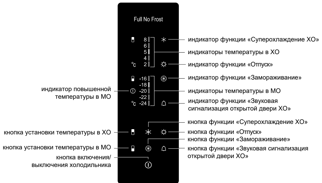
Рисунок 3 — Блок управления
