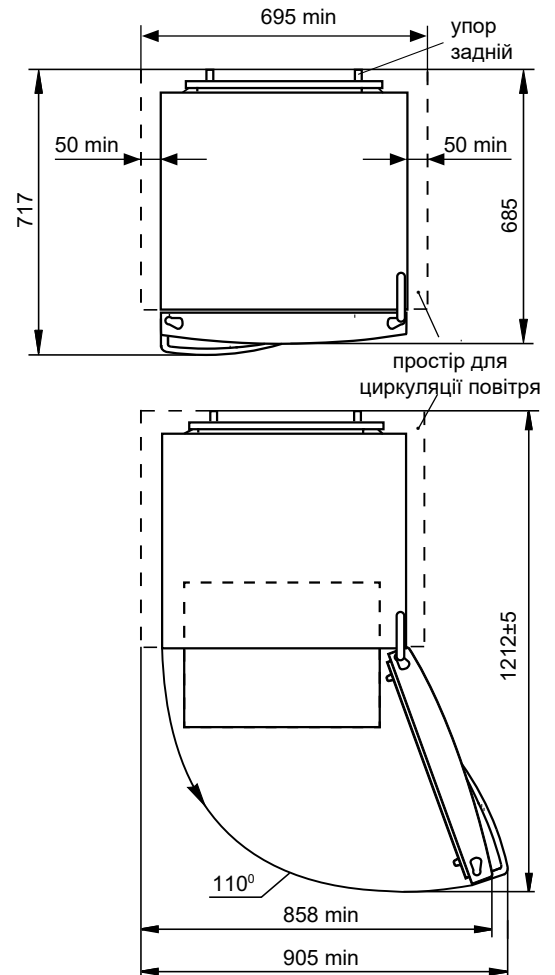
Рисунок 2 — Холодильник (вигляд зверху)
