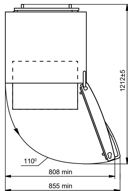
2-сүрөт — Муздаткыч (үстүнөн карагандагы көрүнүш)
