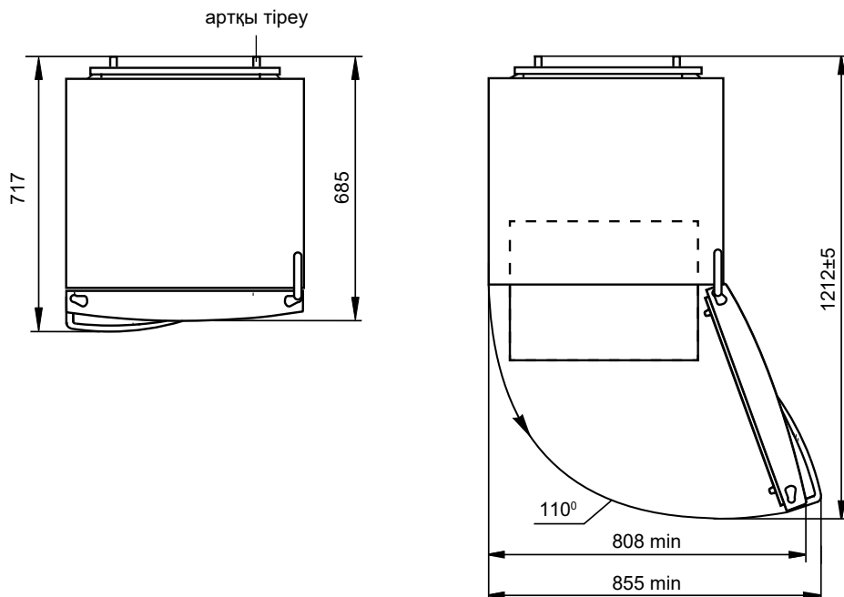
2 сурет — Тоңазытқыш (жоғарыдан көрінетін түр)
