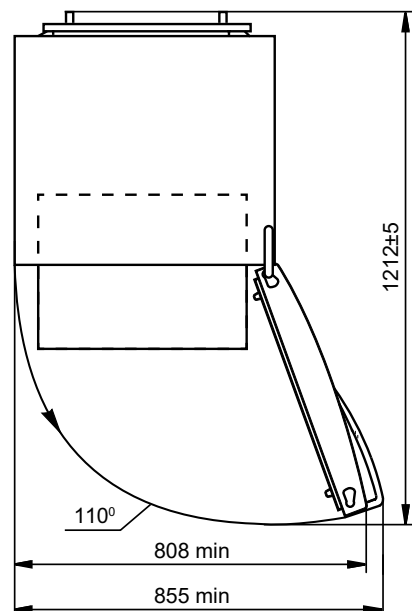
2-rasm – Muzlatgich (yuqoridan ko'rinishi)
