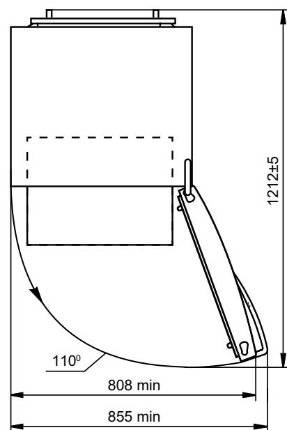
Şəkil 2 — Soyuducu (üstədən görünüşü)
