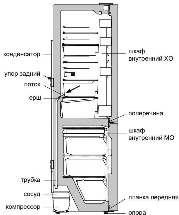
Рисунок 9 – Схема слива талой воды из ХО
