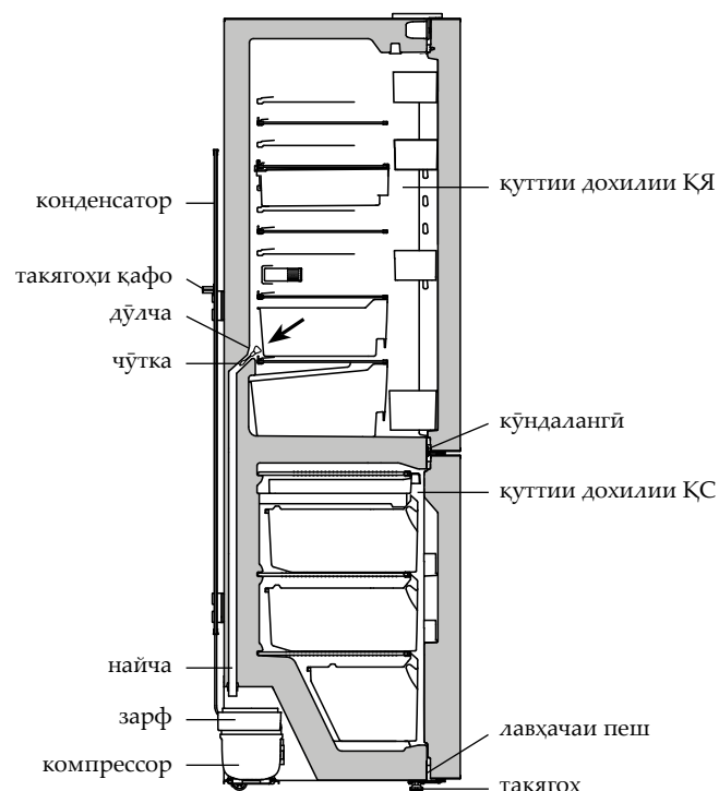
Расми 9 – Нақшаи резини яхоба аз ҚЯ
