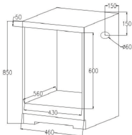
Размеры кухонного модуля
