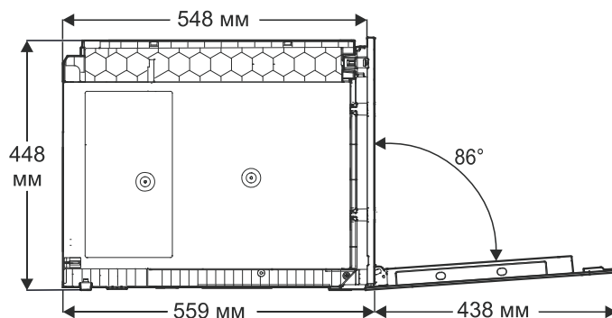
Вид сбоку
