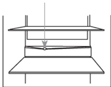
Сливное отверстие.
