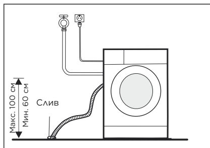
1. Напрямую в канализацию
