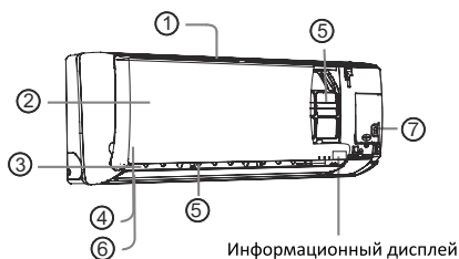
Внутренний блок
