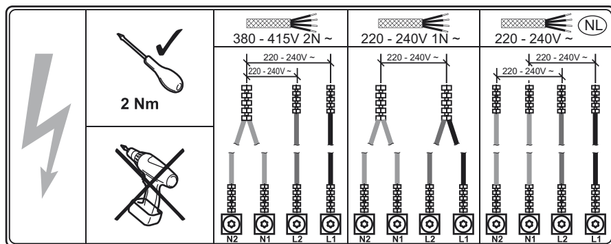
Boje ožičenja
