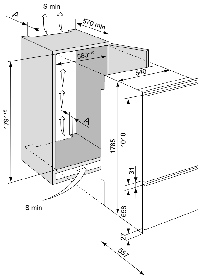
Расми 3 – Сохти васлкунӣ яхдон дар мебел
