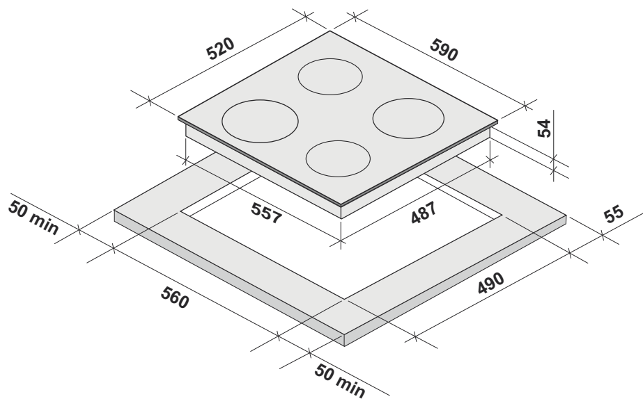
Схема встраивания варочной поверхности FARBE 60 / GENESIS 60
