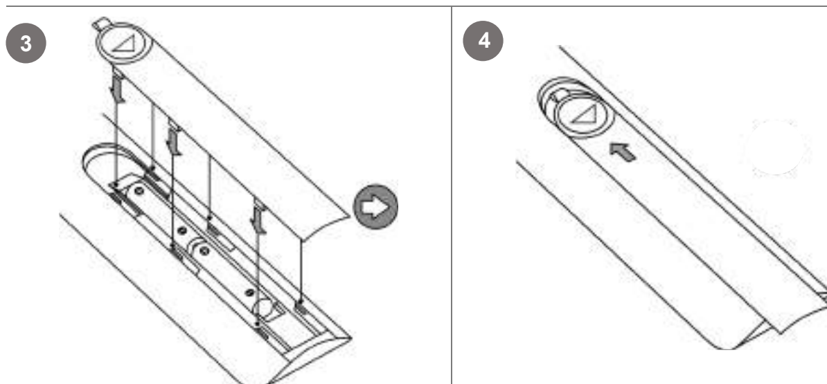
Рисунок 37 – Установка элементов питания в пульт ДУ
