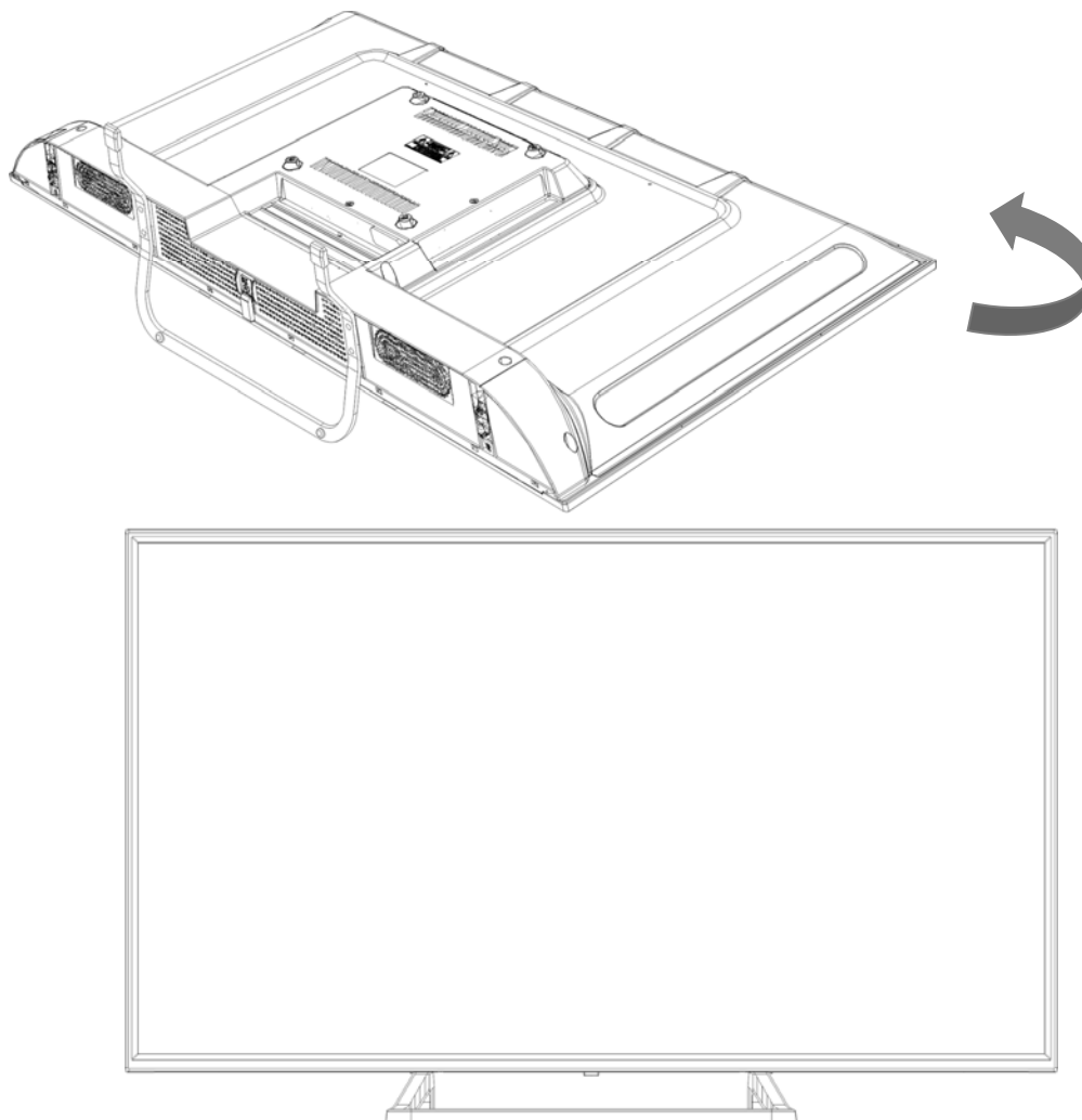
Рисунок 5 – Установка телевизора на поверхность на центральной опоре
