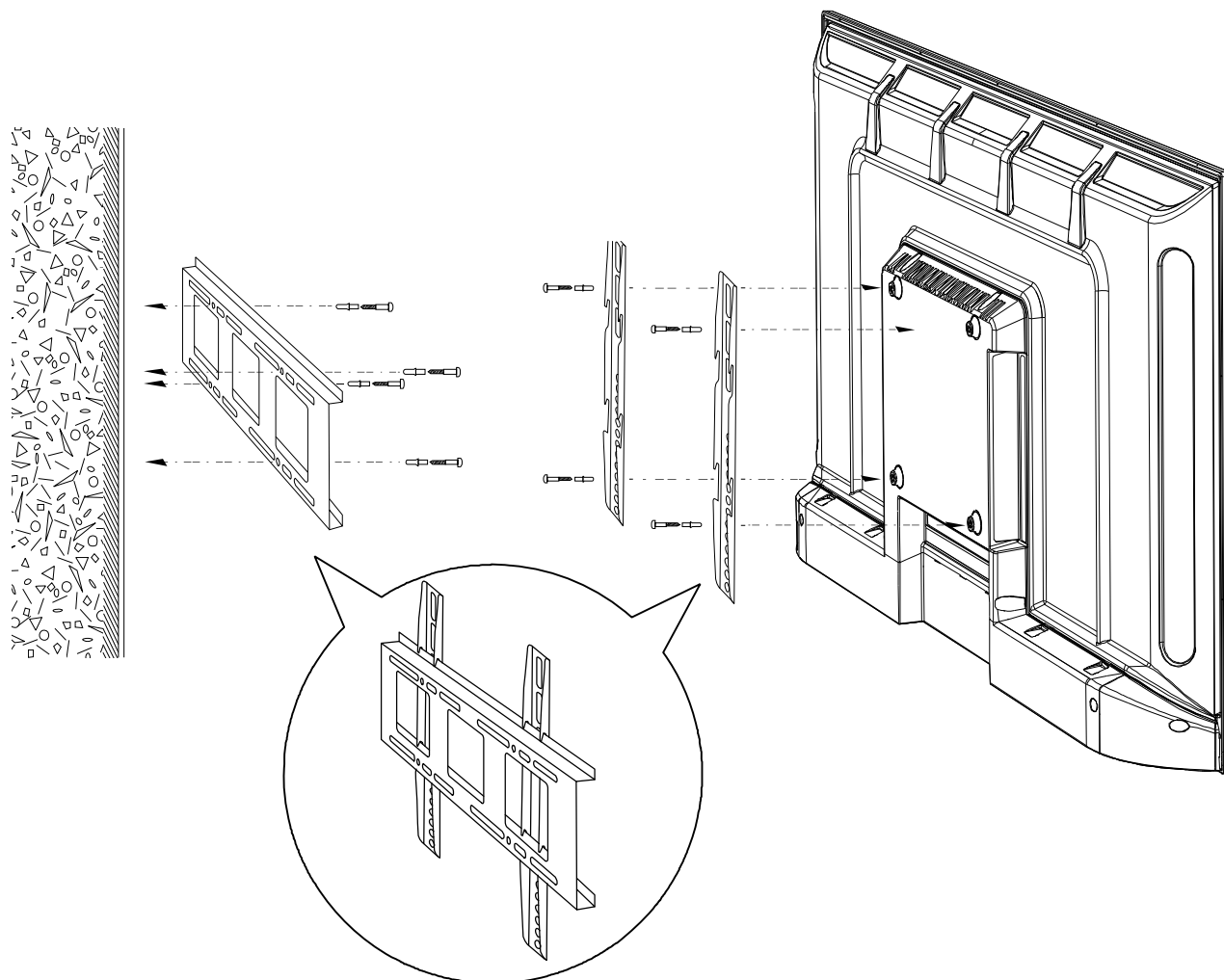
Рисунок 6 – Настенный монтаж телевизора
