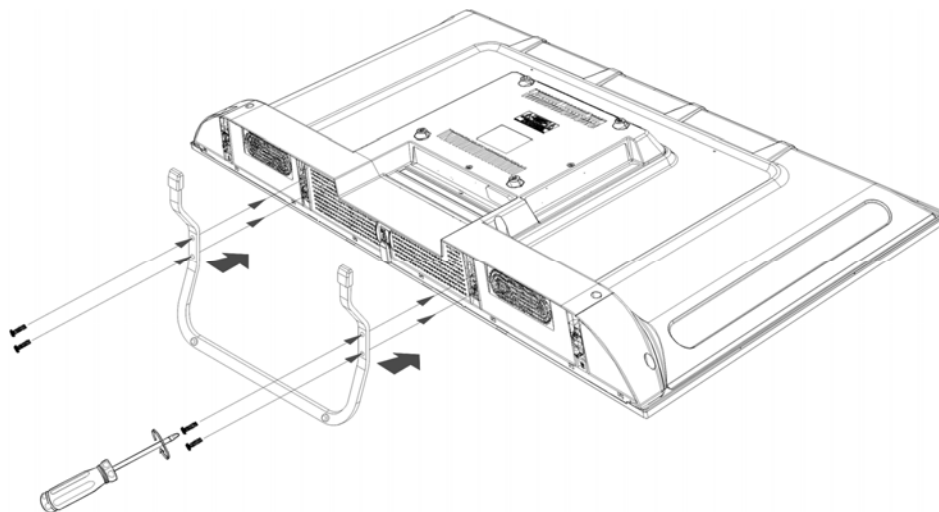
Рисунок 4 – Закрепление центральной опоры
