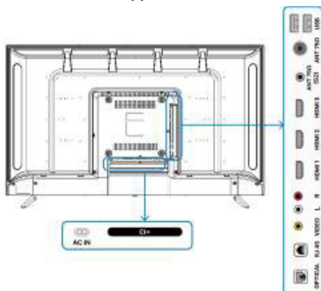
Рисунок 1 – Терминалы задней панели телевизора
