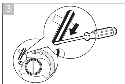
3. Нажмите вниз (в направлении стрелки). Если дверца разблокировалась, индикатор блокировки погаснет.
