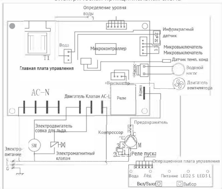
Электрическая принципиальная схема
