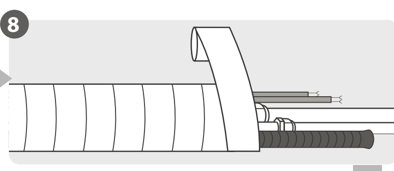
Обвяжите трубопроводы и кабели (не применимо для некоторых регионов в Северной Америке)
