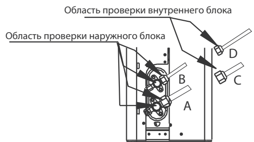
A: Запорный вентиль низкого давления B: Запорный вентиль высокого давления C & D: Конусные гайки внутреннего блока
