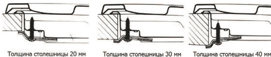
Рис. 6. Положение крепёжных скоб в зависимости от толщины столешницы
