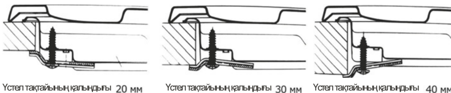
6 сур. Үстел тақтайының қалыңдығына байланысты бекініс қапсырмаларының жайғасымы
