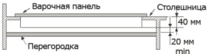
Рис. 7. Положение перегородки
