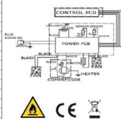
ELECTRIC DIAGRAM Schéma électrique
