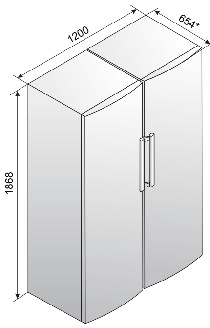
Şəkil 9 – Side by side kombinasiyasının ümumi ölçüləri
