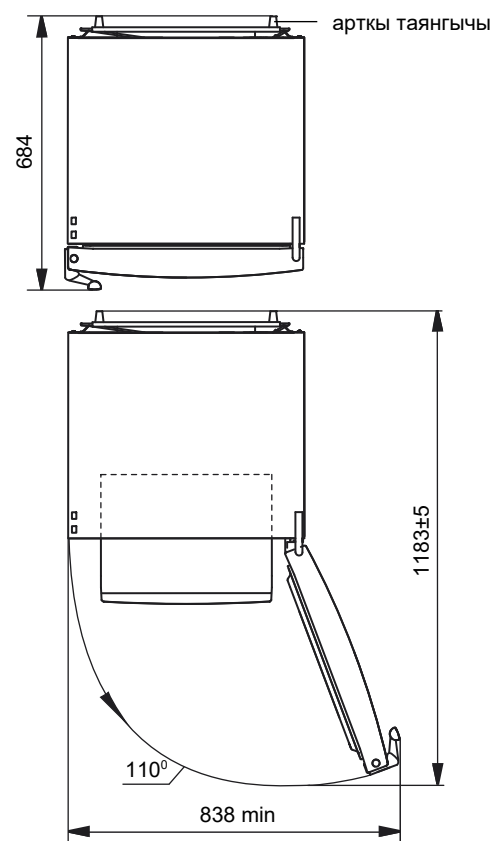
2-сүрөт – Тоңдургуч (устунон корсотулгон)
