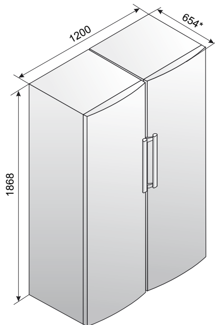
9-сүрөт – Side by side комбинациясынын габариттик өлчөмдөрү
