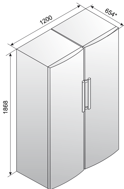
Расми 9 – Ҳаҷми калони комбинатсияи Side by side
