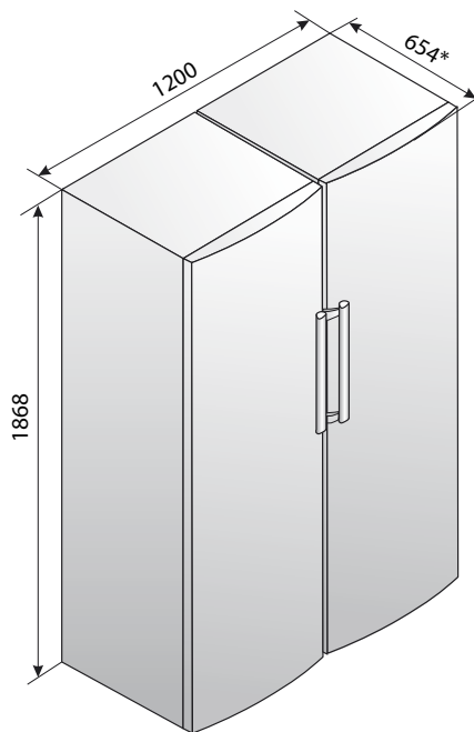
Figura 9 – Dimensiunile generale ale combinației Side by side
