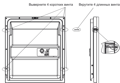
Рис. 5b. Крепление декоративной деревянной панели.
