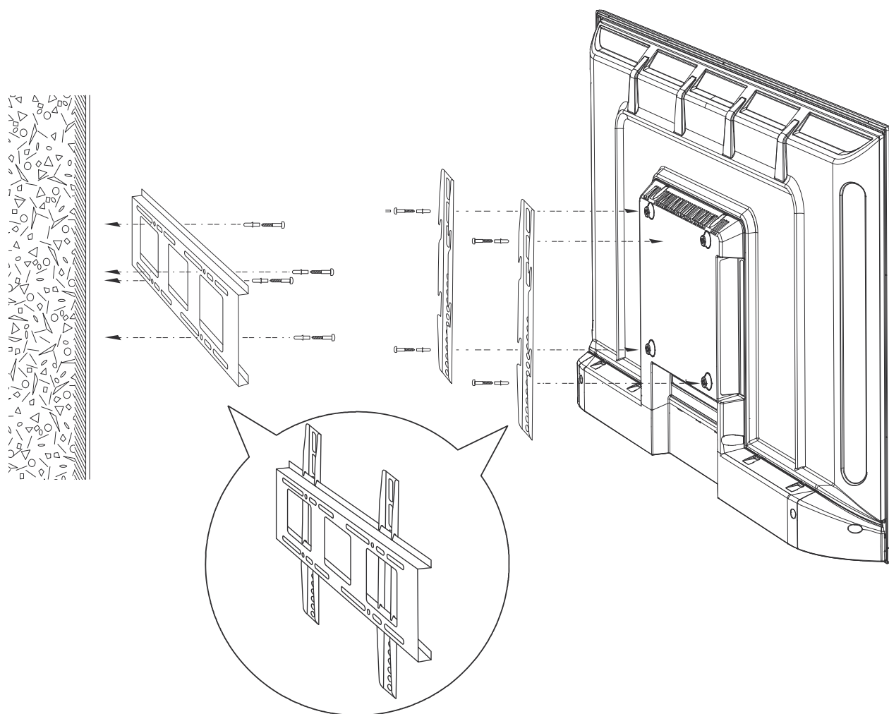
Рисунок 10 – Настенный монтаж телевизора
