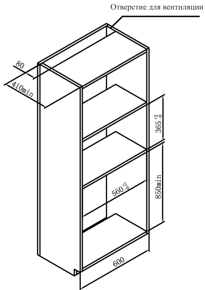
Габариты шкафа
