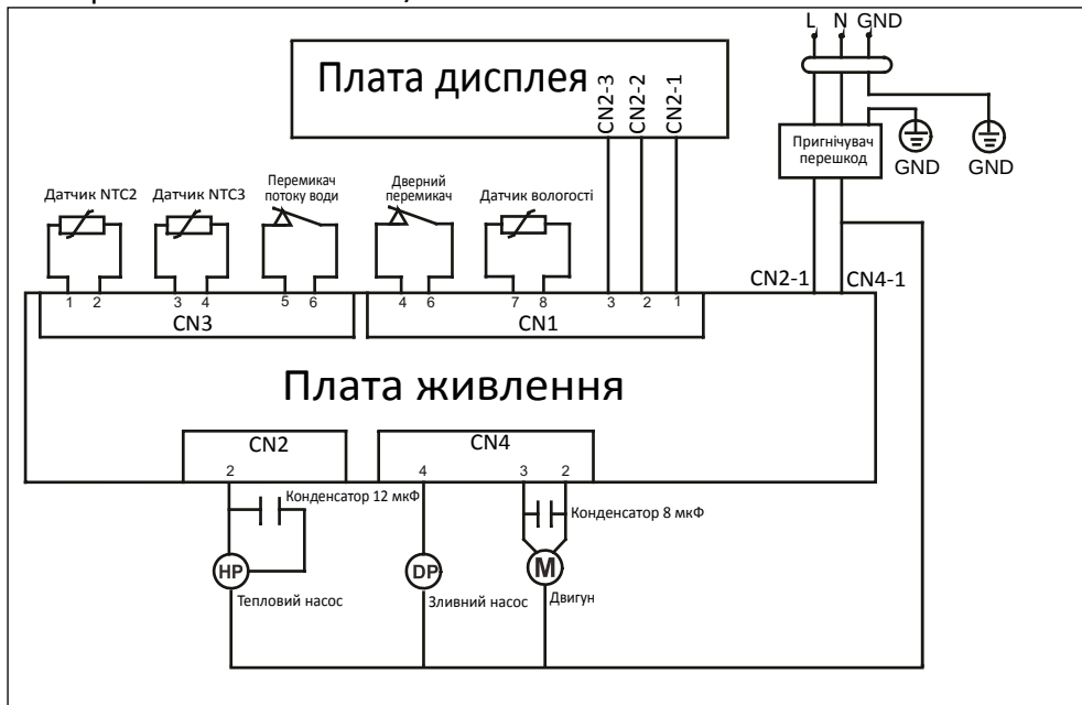
Електросхема HD90-A2959/HD90-A2959S:
