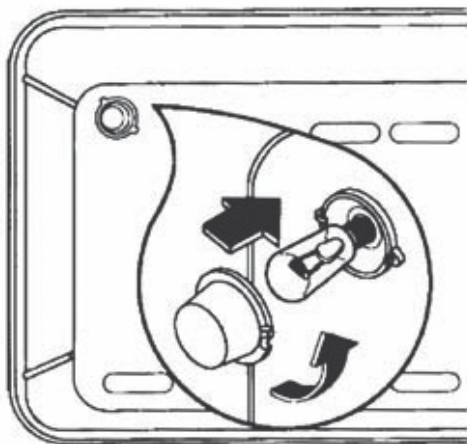
Рис. 13. Замена лампы
