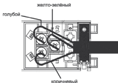
Рис. 12. Схема подключения
