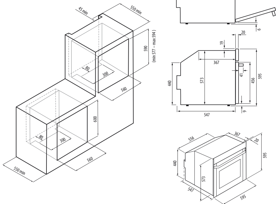
Рис. 9. Схема встраивания духового шкафа
