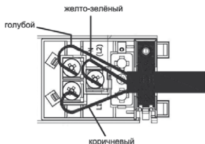
Рис. 11. Схема подключения
