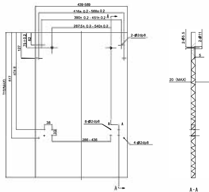
Рис. 3. Единицы измерения – мм
