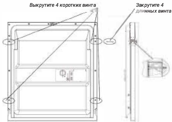
Рис. 5 Установка внешней панели
