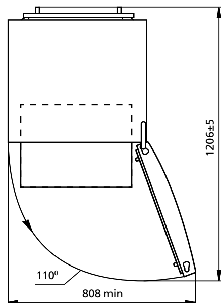
Тасвири 2 — Яхдон (намо аз боло)
