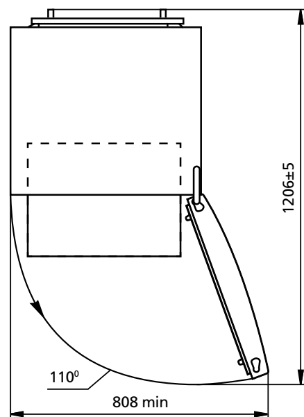
2-rasm – Muylatgich (yuqoridan ko'rinishi)
