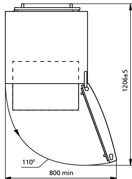
Şəkil 2 — Soyuducu (üstdən görünüşü)
