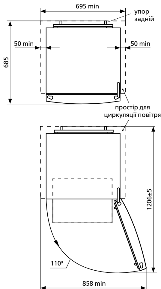
Рисунок 2 — Холодильник (вид зверху)
