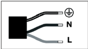
Провода: Желто-зеленый → Заземление (⏏) Синий → Нейтральный (N) Коричневый → Фаза (L)
