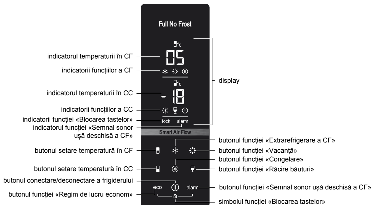
Figura 3 – Panoul de control
