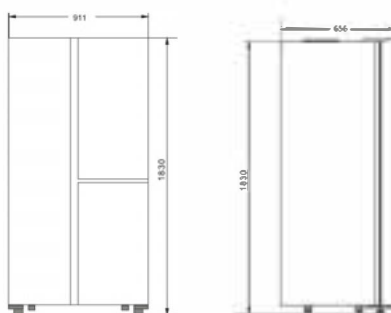
Модель CS6073FV
