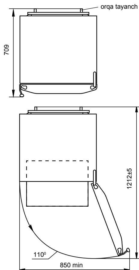
2-rasm – Sovutgich (tepadan ko'rinishi)
