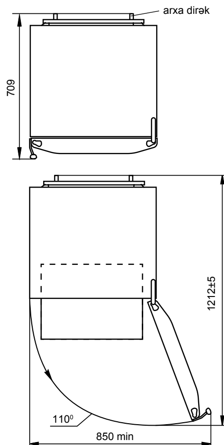
Şəkil 2 – Soyuducu (üstədən görünüşü)
