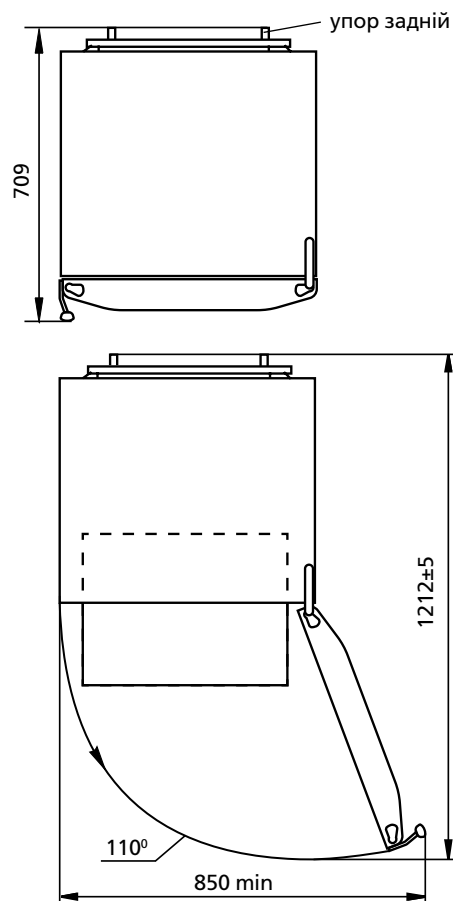
Малюнок 2 — Холодильник (вигляд зверху)
