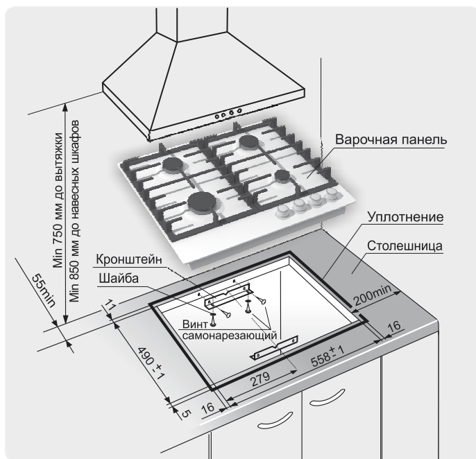
Рис. 5 МОДЕЛЬ ПВГ 1214; -01
