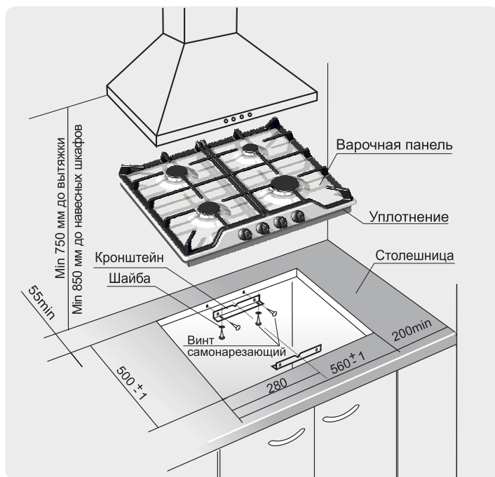
Рис. 4 МОДЕЛЬ ПВГ 1212; -01
