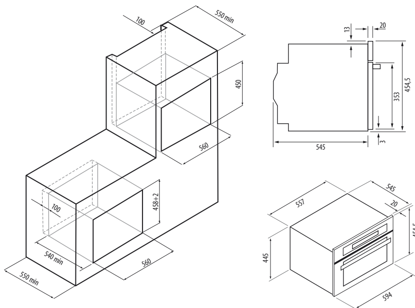
Схема встраивания духового шкафа.
