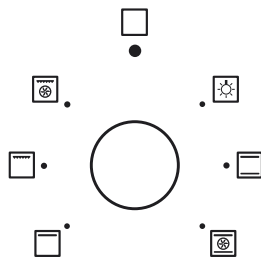
Рис. 3. Переключатель режимов работы духового шкафа
