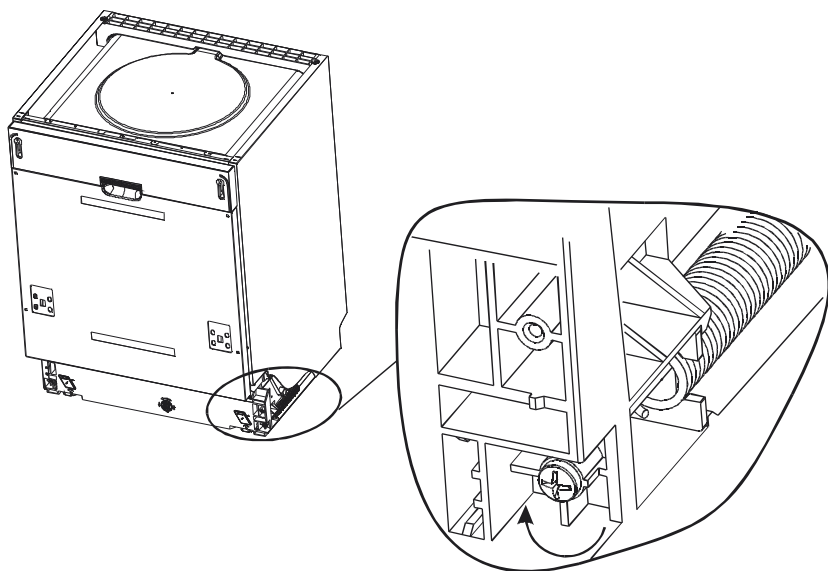
Рис. 4b. Крепление декоративной деревянной панели.
