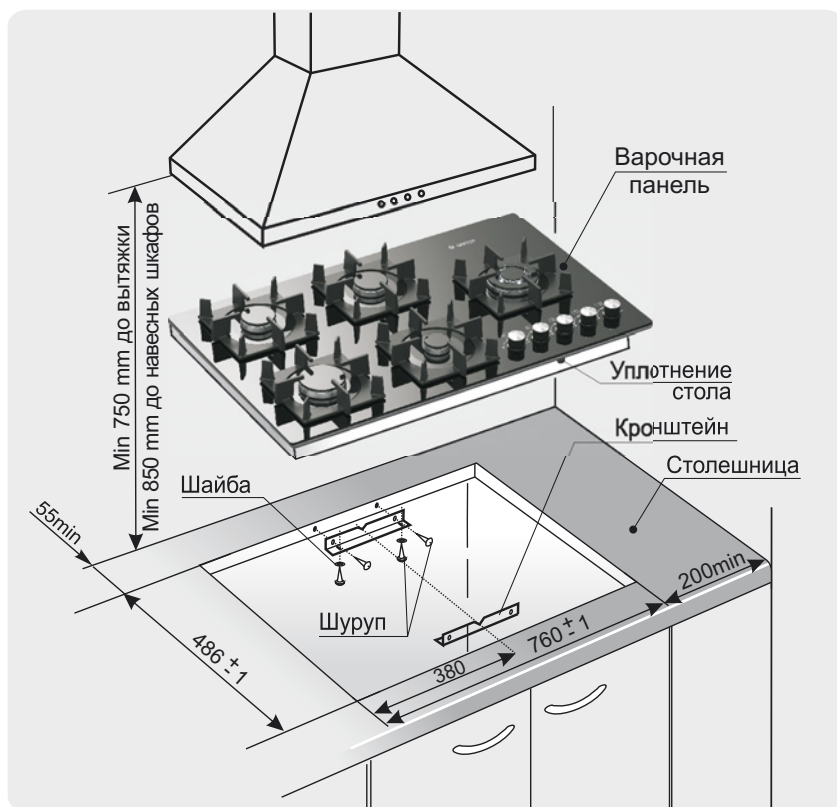
Рис. 5 МОДЕЛЬ ПВГ 2341
