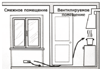
Рис. 3. Устройство вентиляции через смежное помещение
