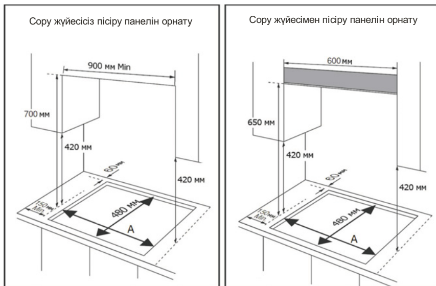
5 сур. Аспап орнатуға арналған орынды дайындау (А – өлшемі, 3 кест. қар.)
