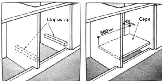
8 сур. Тұмшاپеш астына арналған түпқойма нұсқалары
