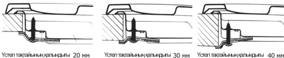
6 сур. Үстел тақтайының қалыңдығына байланысты бекініс қапсырмаларының жайғасымы
