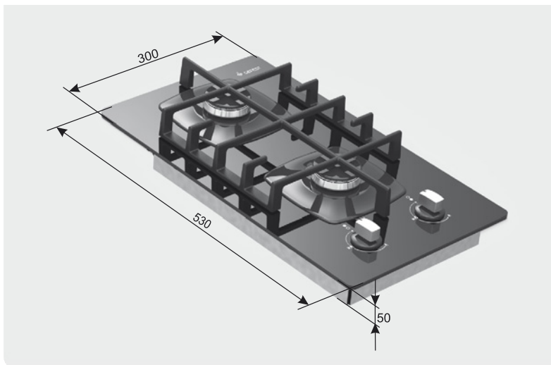
Рис. 2 МОДЕЛЬ ПВГ 2002
