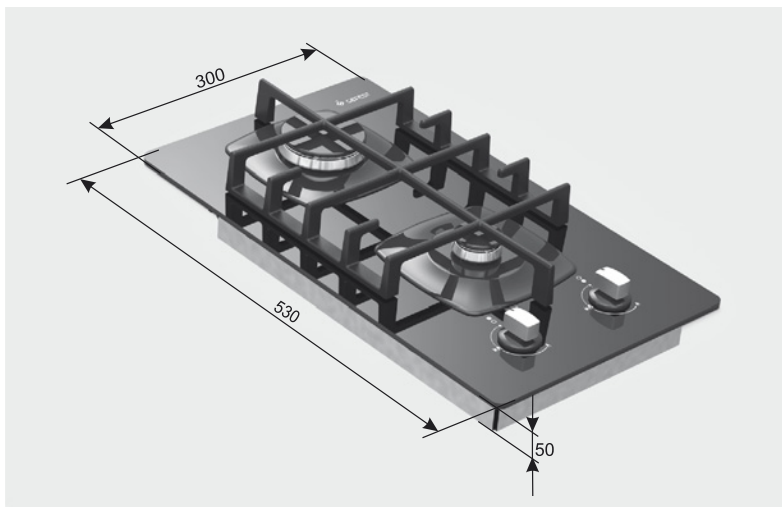
Рис. 3 МОДЕЛЬ ПВГ 2003
