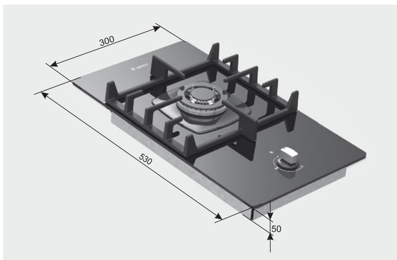
Рис. 1 МОДЕЛЬ ПВГ2001
