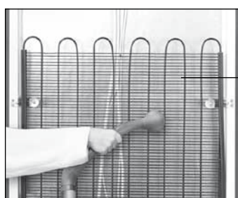
конденсатор
