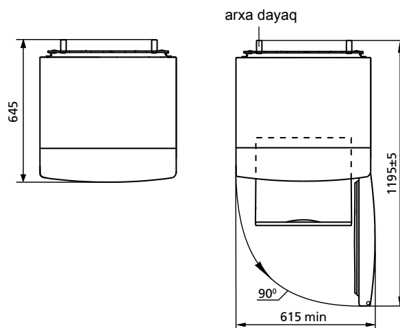
Şəkil 2 – Soyuducu (yuxarıdan görünüş)
