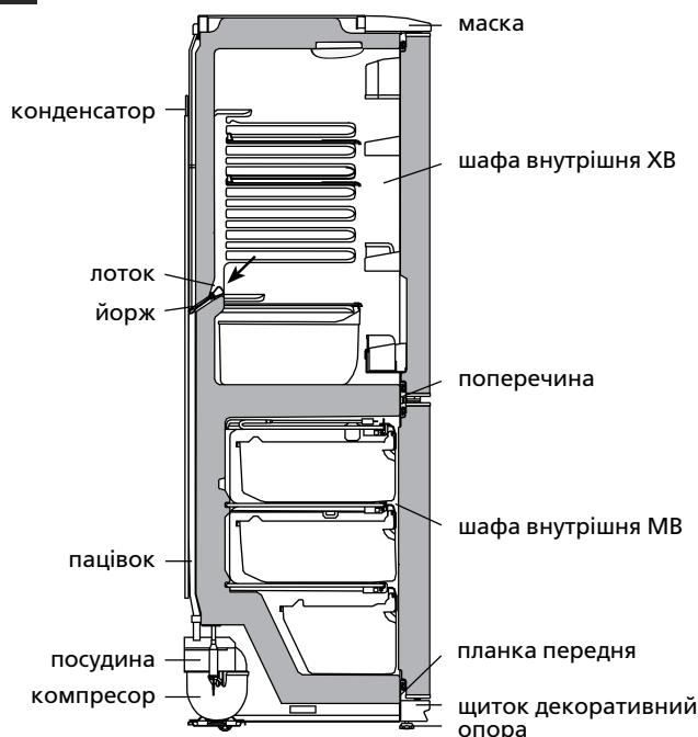
Рисунок 4 – Схема зливу талої води із ХВ
