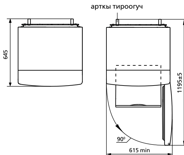
Сурот 2 – Муздаткыч (устунон корунушу)
