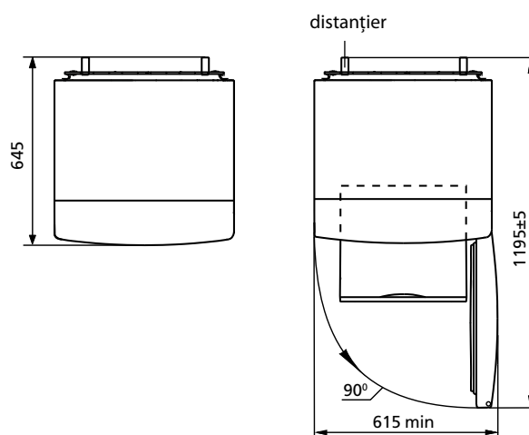
Figura 2 – Frigider (vedere de sus)
