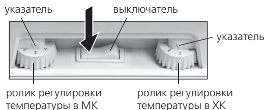
Рисунок 10 — Схема переключения режимов в холодильнике двухкомпрессорном или в однокомпрессорном холодильнике с клапаном
